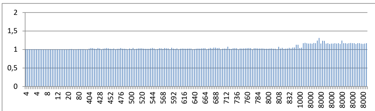
39. ábra Az 1 processzorhoz képest Amdahl képlete alapján számított gyorsulás 4 processzor használata esetén. A vízszintes tengelyen a 4 processzor által együtt számított szabálybázisok száma látható.
