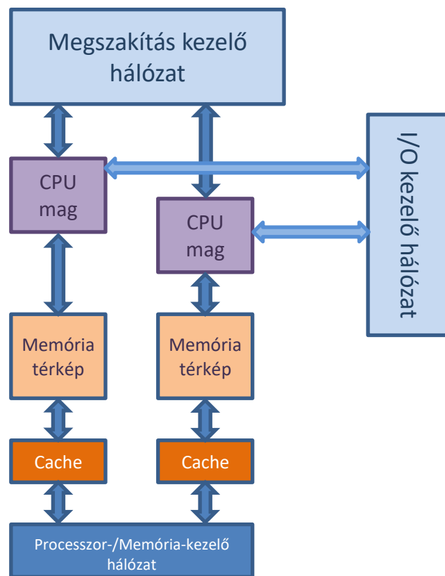
22. ábra Szorosan csatolt többprocesszoros rendszer, egyszerűsített ábra
