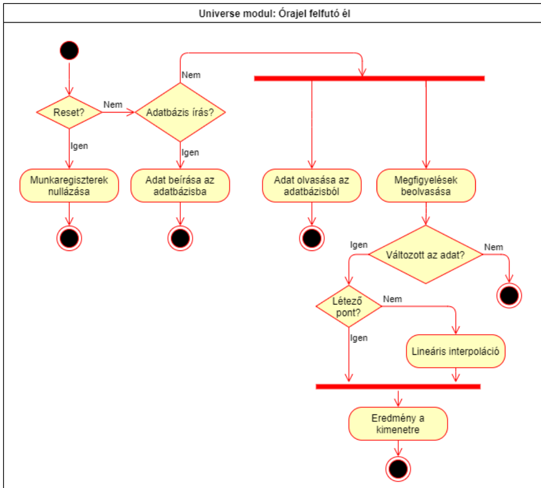
48. ábra A FIVE Universe moduljának működési vázlatja
