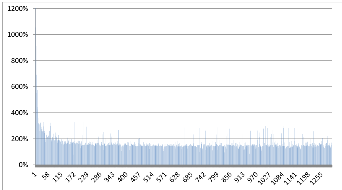
29. ábra A nem gyorsítótárazott adattal végzett számítások idejének hossza a gyorsítótárazott adattal végzett időkhöz képest 1 processzormagon. A grafikon vízszintes tengelyén a számításban résztvevő szabályok száma látható. Maximum érték: 1844%, átlag: 163%
