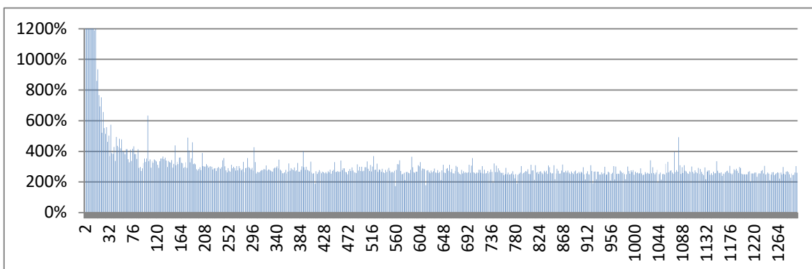
35. ábra 2 CPU használata esetén a nem gyorsítótárazott adatokkal végzett vizsgálatok hosszabb ideig tartanak. Az x tengely a számításban részt vevő szabálybázisok számát jelzi. Átlag: 275 % Maximum: 2899 %
