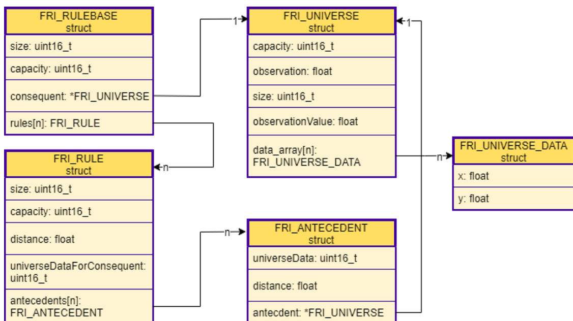
10. ábra Az \mu FRI könyvtár adattároló struktúrájának ábrázolása
