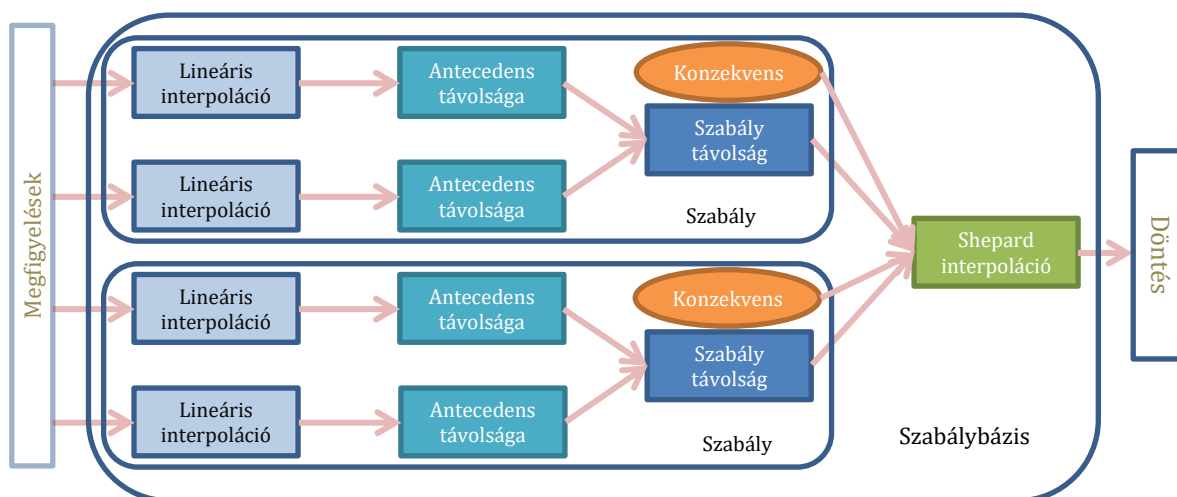
11. ábra A \mu FRI könyvtár számítási lépései
