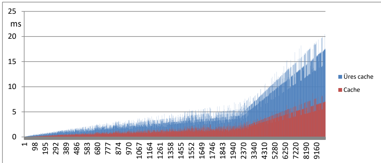
33. ábra A számítási idő változása 2 CPU esetén a szabálybázis számának növekedése függvényében. A vízszintes tengely az 1 CPU-ra eső szabálybázisok számát mutatja
