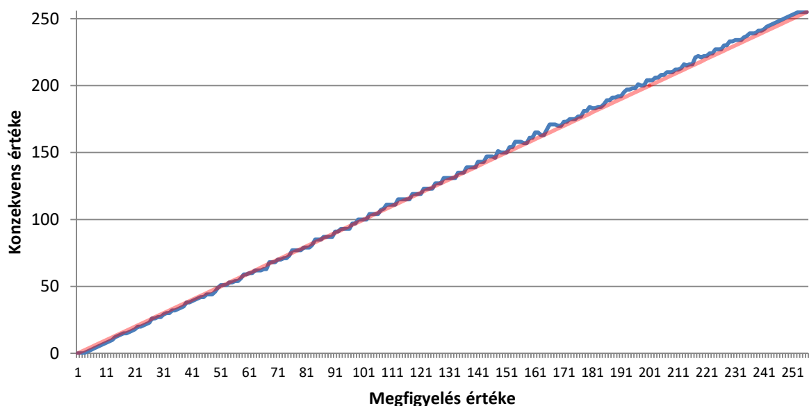
59. ábra A linearitás vizsgálata. A piros vonal az elvárt értéket, a kék vonal a számított értéket jelöli. Az elvárt értéket a \mu FRI C nyelvű megvalósítása számolta.
