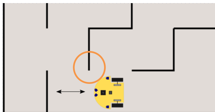
71. ábra Fals folyosó érzékelés a FIVE alapú osztályozónál
