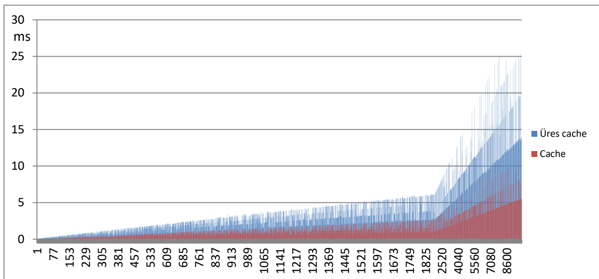
32. ábra A számítási idő változása 1 CPU esetén a szabálybázis számának növekedése függvényében. A vízszintes tengely a szabálybázisok számát mutatja
