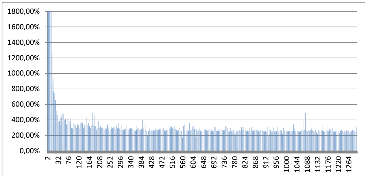
30. ábra A nem gyorsítótárazott adattal végzett számítások idejének hossza a gyorsítótárazott adattal végzett időkhöz képest 2 processzormagon. A grafikon vízszintes tengelyén a számításban résztvevő szabályok száma látható. Maximális érték: 2899 %, átlagérték: 275 %
