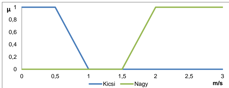
3. ábra Ritka partíció példa
