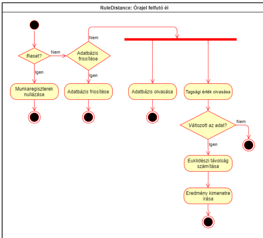
52. ábra A RuleDistance modul működési vázolata
