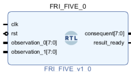
46. ábra Az FRI_FIVE befoglaló modul portjai
