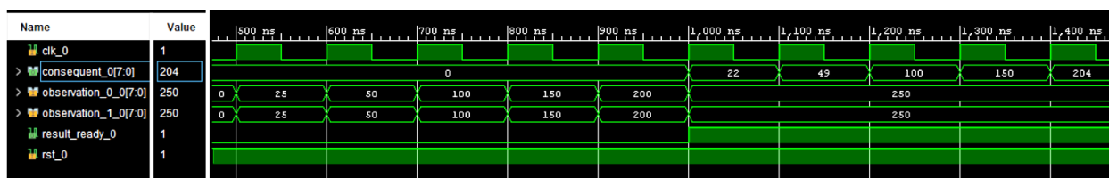
58. ábra Pipeline működést szemléltető szimuláció
