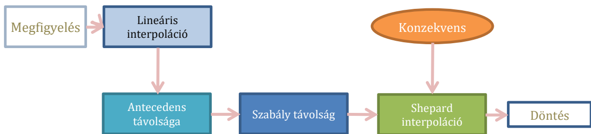
9. ábra A FIVE módszer számítási lépései
