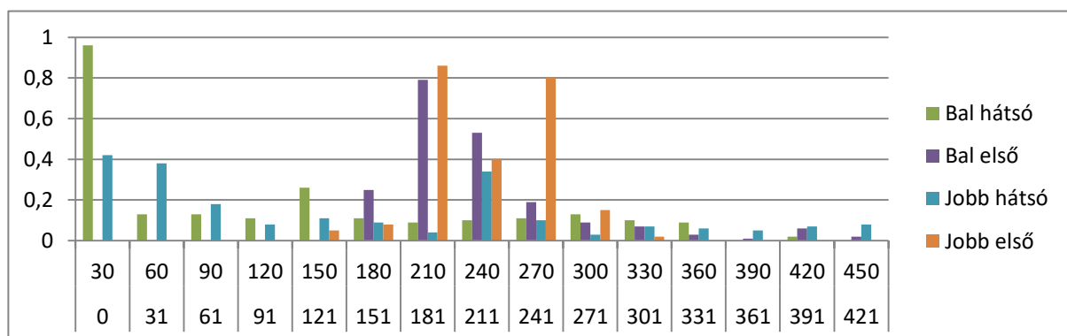
68. ábra Az összes érzékelő klaszterezett adatainak valószínűségei a g mintázat esetén
