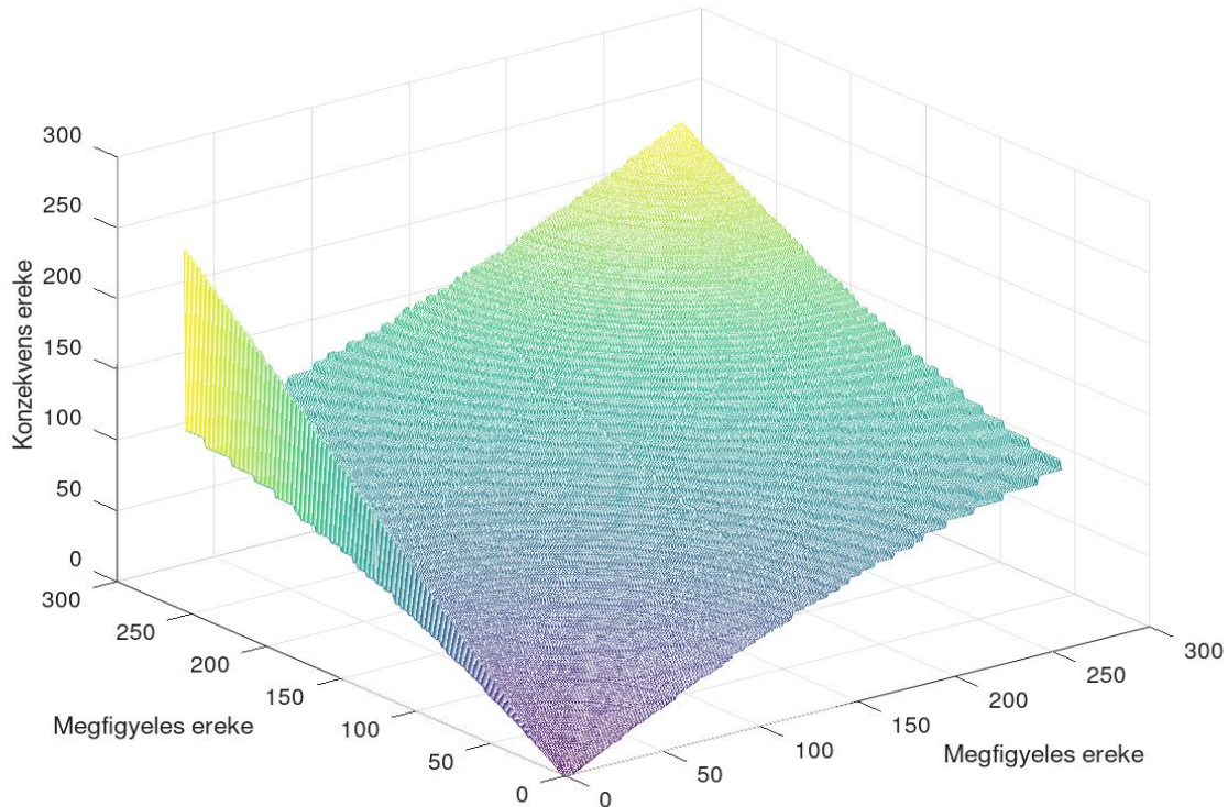
61. ábra Szimulációs eredmények a teljes értelmezési tartományra
