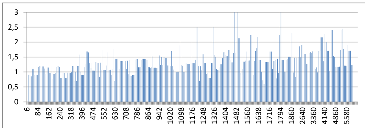
41. ábra Az 1 processzorhoz képest össz számítási idők alapján számított gyorsulás 3 processzor használata esetén. A vízszintes tengelyen a 3 processzor által együtt számított szabálybázisok száma látható. Átlag: 1,5 Medián: 1,25 Módusz: 1,4
