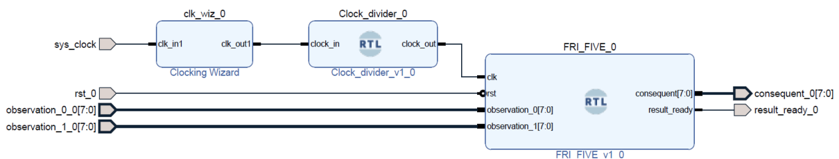
55. ábra A mintában megadott rendszer diagramja
