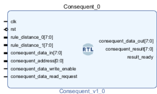
53. ábra A Consequent modul blokk-rajza
