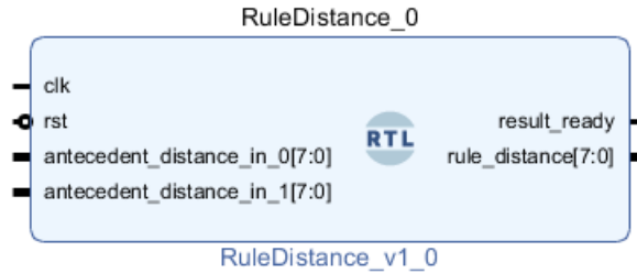
51. ábra A RuleDistance modul portjai
