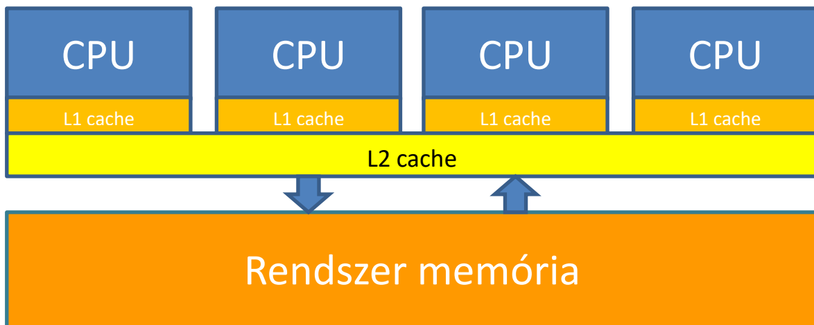
24. ábra Többprocesszoros cache megoldás
