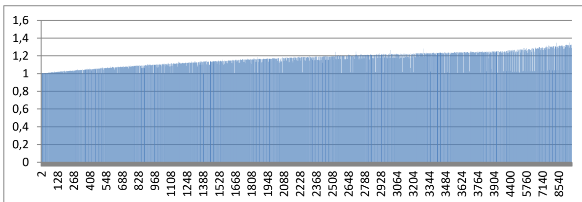
37. ábra Az 1 processzorhoz képest Amdahl képlete alapján számított gyorsulás 2 processzor használata esetén. A vízszintes tengelyen a 2 processzor által együtt számított szabálybázisok száma látható.
