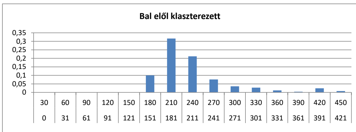
67. ábra Felül a klaszterezés előtti értékek valószínűségei alul pedig a klaszterezés után az egyes tartományok valószínűségei a bal első érzékelő esetén, amikor van előtte fal
