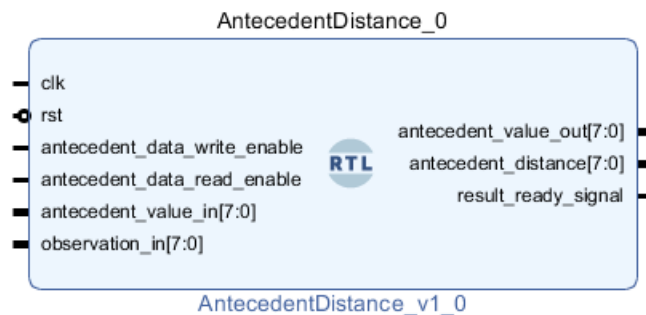
49. ábra Az AntecedentDistance modul blokk-rajza
