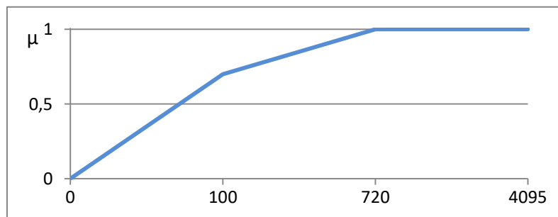
70. ábra A „leftBack” univerzum grafikonja (a vízszintes tengely az ADC - Analog-Digital Converter - értéket veszi fel)
