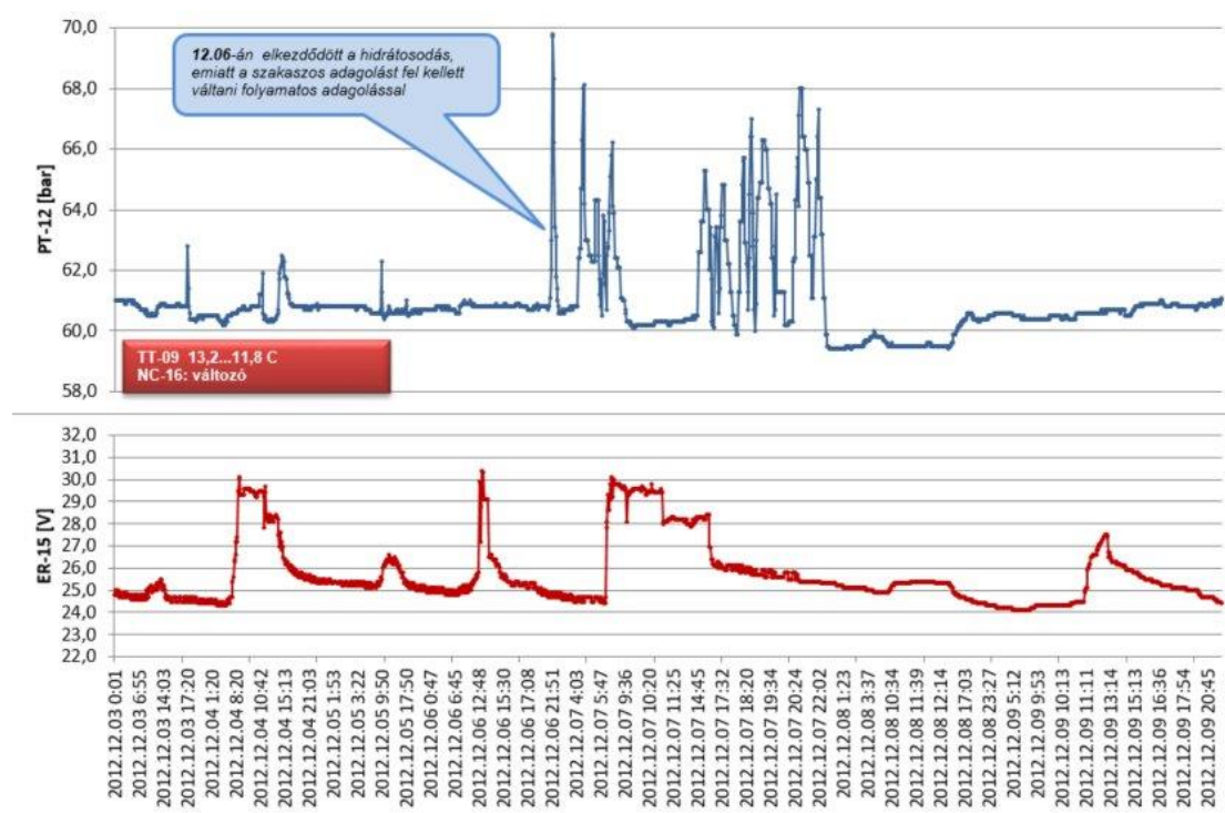
43. ábra Adatok kiértékelése
