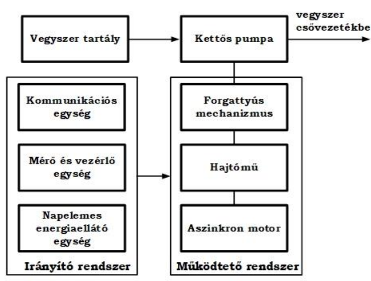
34. ábra A vegyszeradagoló blokkvázlatos felépítése
