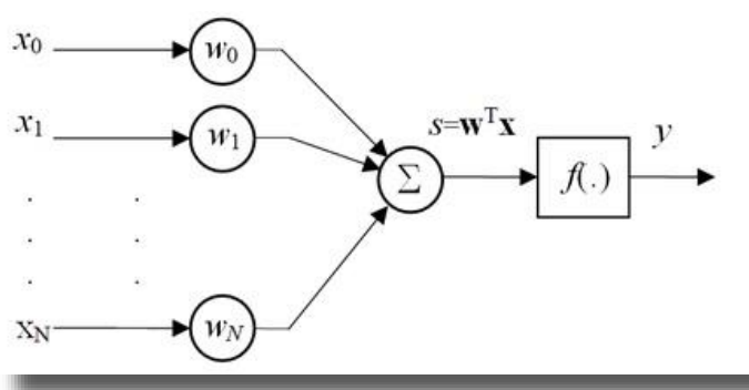
22. ábra Neuron matematikai modell [46]
