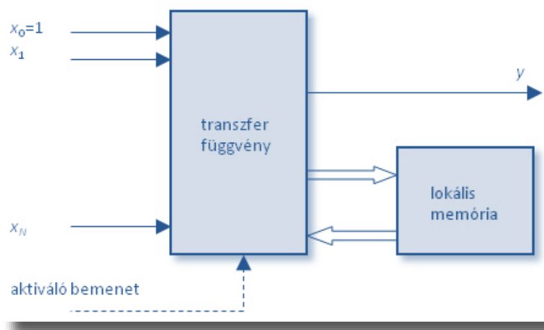
21. ábra Neuron elvi felépítése [36]
