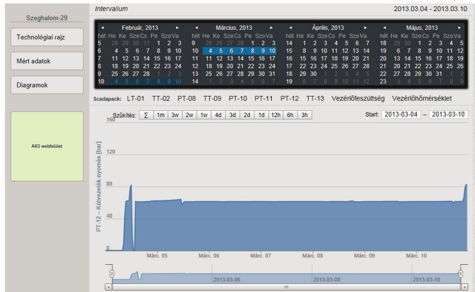
42. ábra Adatok megjelenítése
