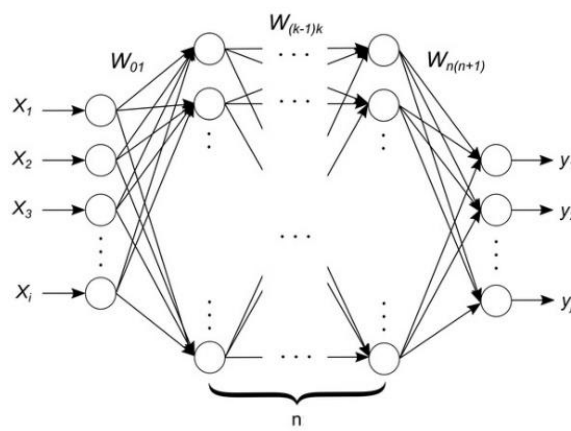
26. ábra n rétegű perceptron [40]
