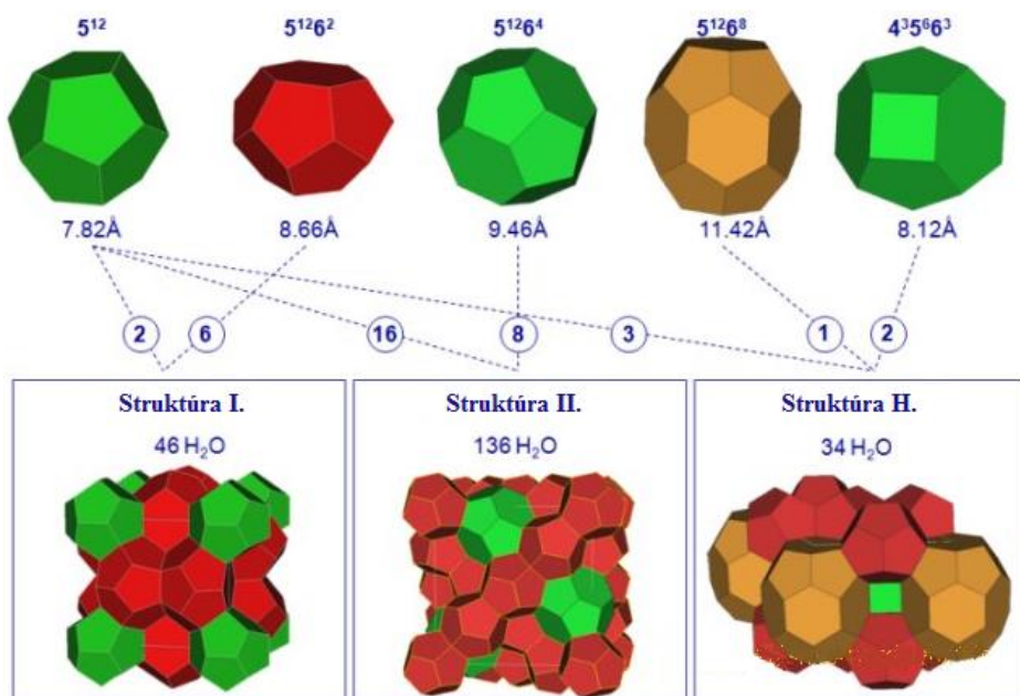
3. ábra Hidrát struktúrák [10]
