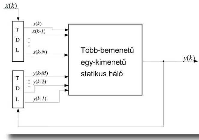
27. ábra Időfüggő hálózat [46]
