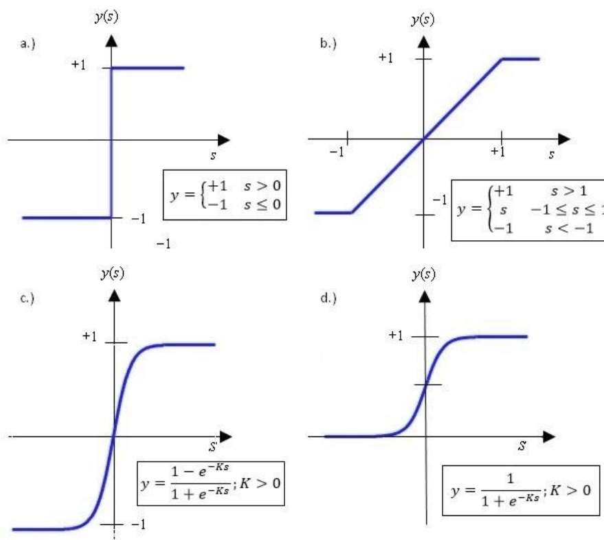
23. ábra Tipikus nemlineáris függvények [36]
