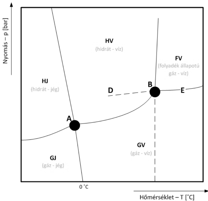
2. ábra Fázishatár görbe [4]
