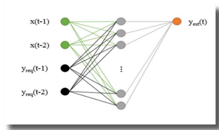
29. ábra NNARX modell
