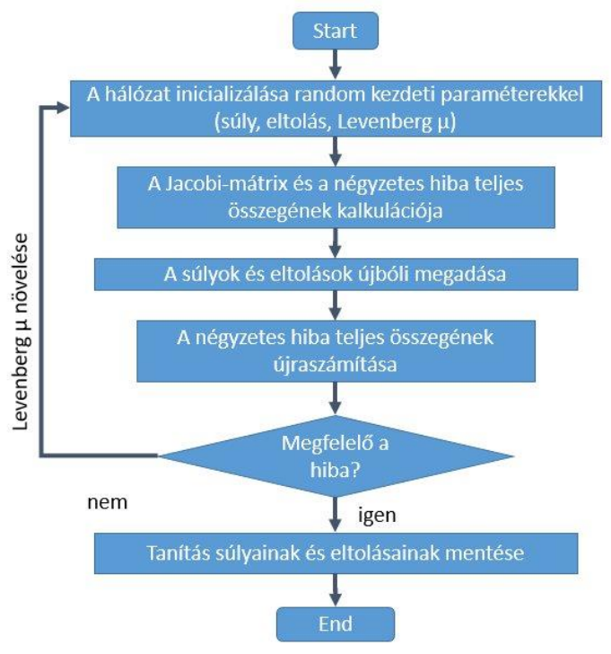
31. ábra Levenberg–Marquardt eljárás [40]
