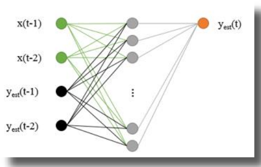
28. ábra NNOE modell
