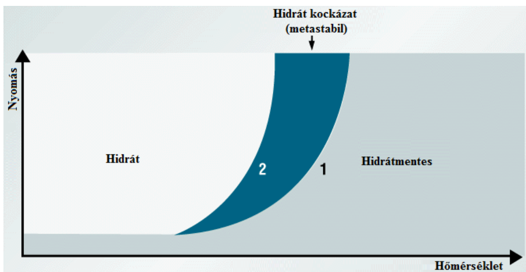
5. ábra Hidrátosodási zónák [12]
