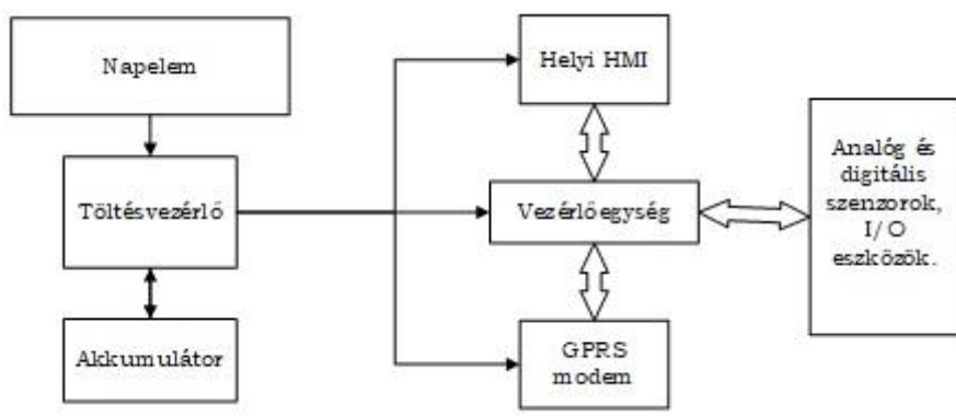
36. ábra A napelemes rendszer
