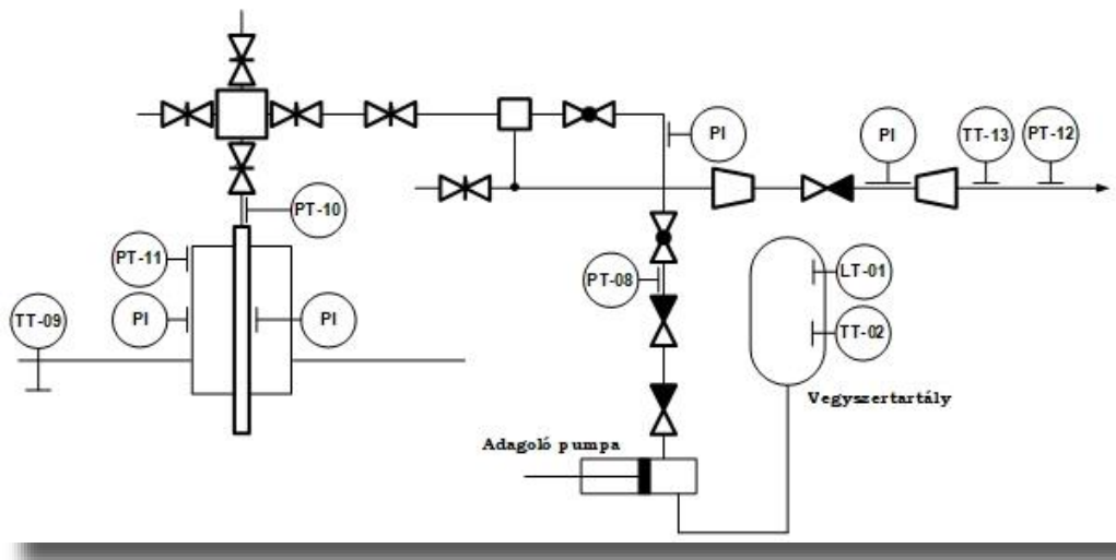
38. ábra A kútkörzeti műszerezettség
