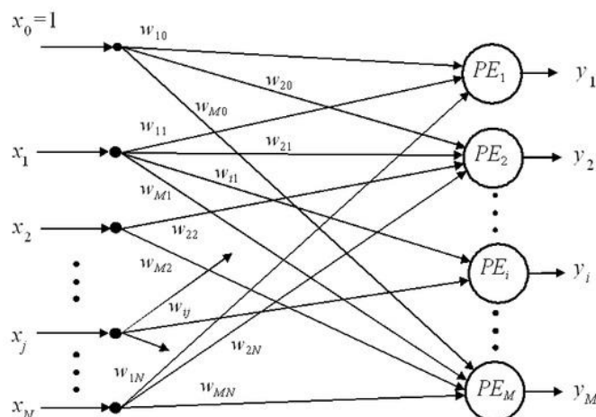
24. ábra Előrecsatolt hálózat [36]
