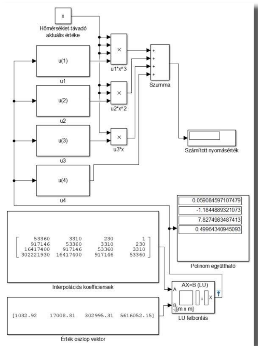
11. ábra Nyomásérték meghatározó modell
