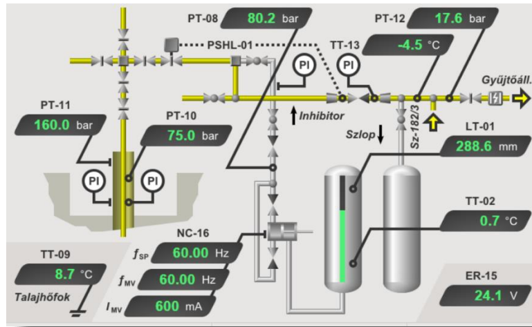
41. ábra Webfelület
