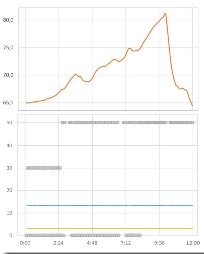
44. ábra Adathalmaz
