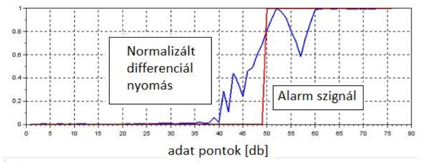
30. ábra Riasztási szint – 75%
