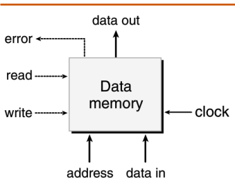
1.15. ábra. RAM memória működése.
