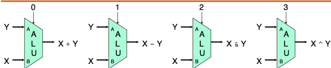
1.11. ábra. Aritmetikai és logikai egység (ALU). A funkció választó bemenet értékétől függően, az áramkör a négy különböző aritmetikai és logikai művelet egyikét végzi el.
